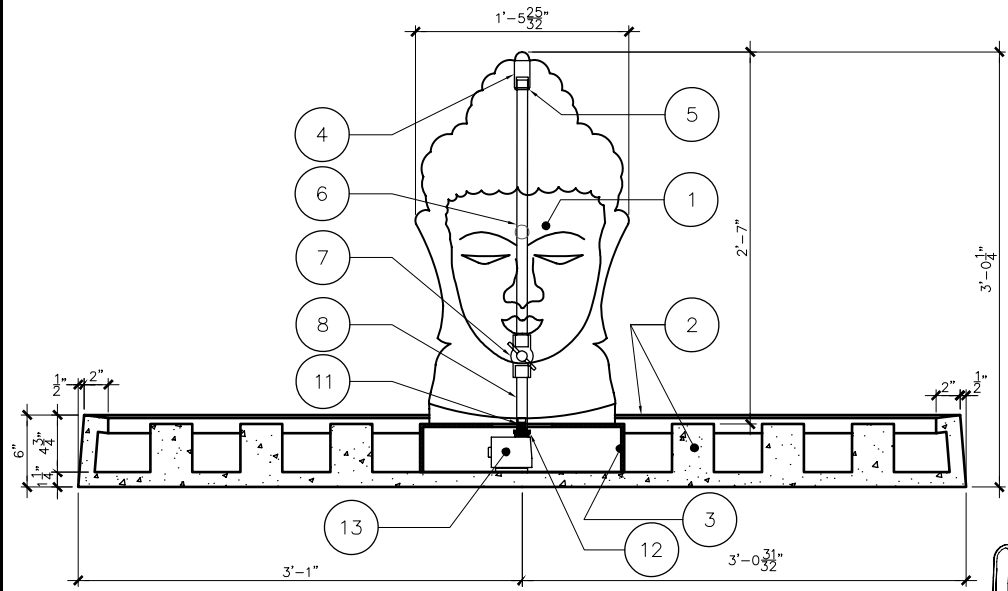
2 ELEVATION SCALE: 3/4"=1'-0"
