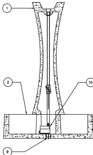
4 SECTION SCALE: 3/4"=1'
