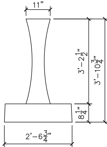
2 ELEVATION SCALE: 1/2"=1'
