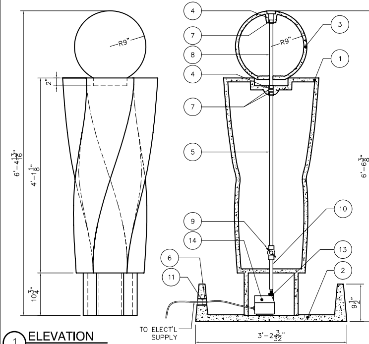
2 SECTION SCALE: 1/2"=1'
