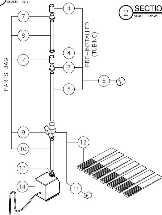
1 ELEVATION SCALE: 1/2"=1'
